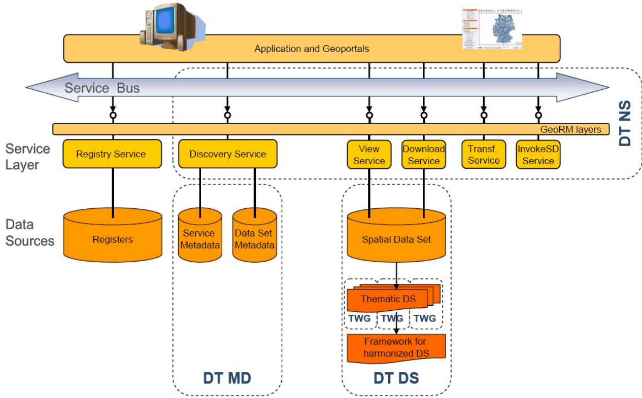
Şekil 1: INSPIRE teknik mimarisi (INSPIRE, 2007)
