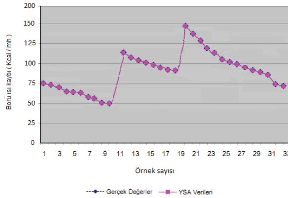
Şekil 14. Yalıtımlı boru yapısı için ısı kaybının YSA verileri ile gerçek verilerin karşılaştırılması
