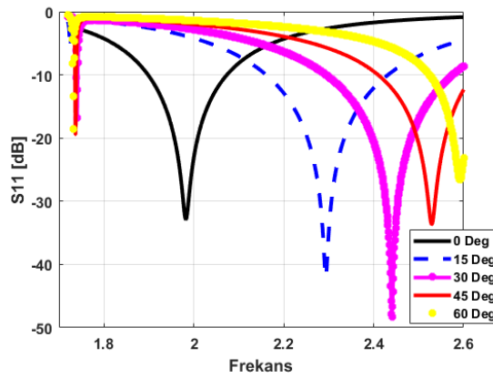
Şekil 4. Açısally döndürülen yamanın yansıma grafiğı
