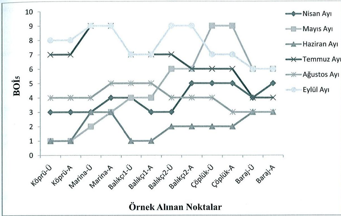
Şekil 5. Borçka Baraj Gölünde BOI 5 aylara göre değişimi
