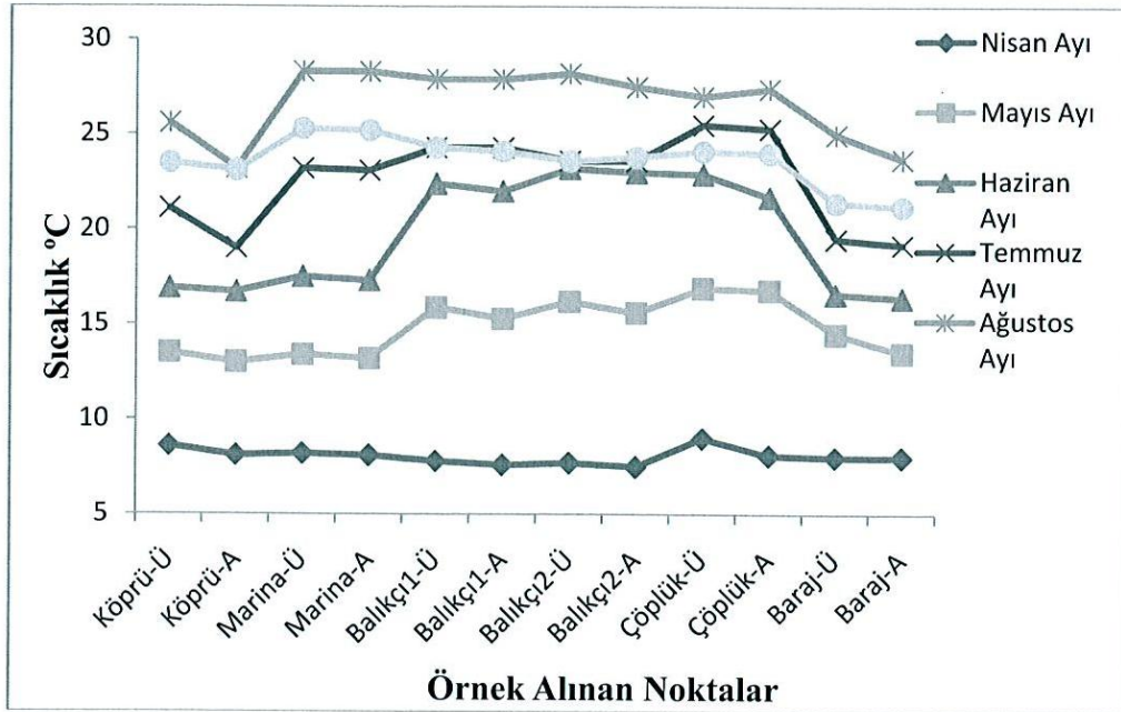
Şekil 2. Borçka Baraj Gölünde sıcaklığın aylara göre değişimi
