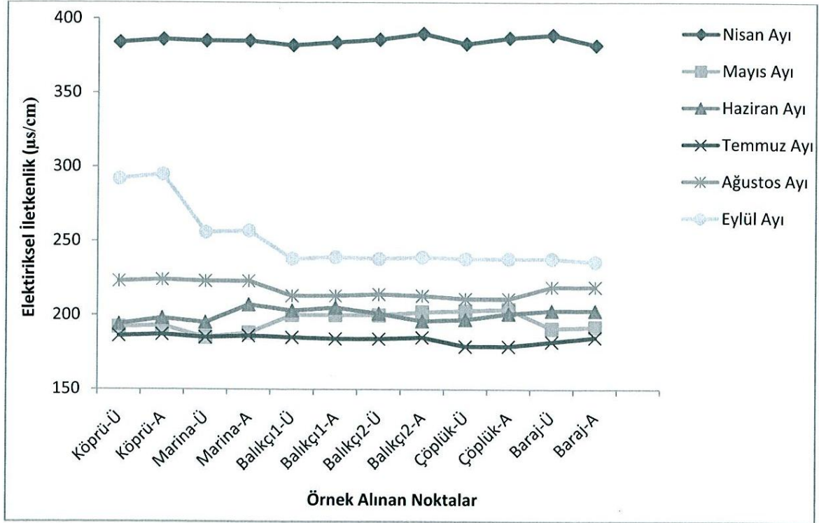
Şekil 4 . Borçka Baraj Gölünde elektriksel iletkenliğin (µS/cm) aylara göre
