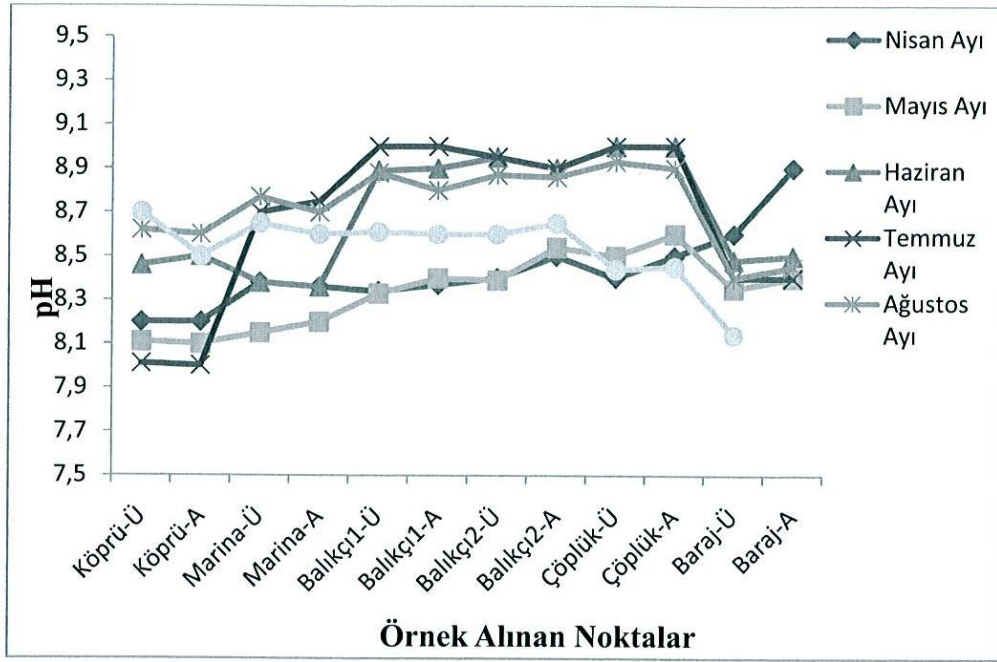
Şekil 1. Borçka Baraj Gölünde pH'nın aylara göre değişimi
